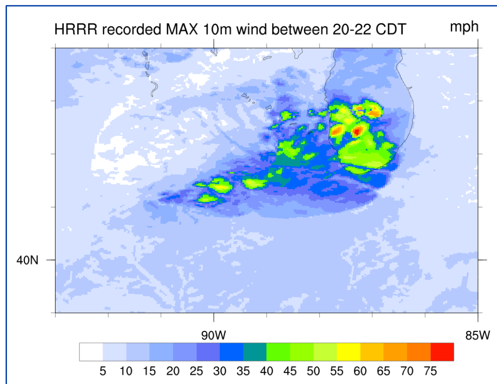
HRRR
